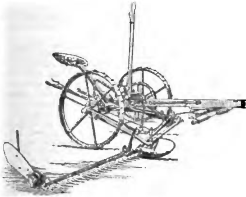
FIG. 2.—Mower (side view).
