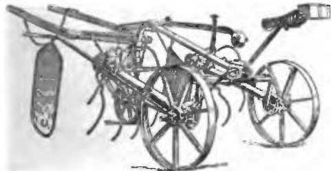
FIG. 3.—Swathe-turner. (Blackstone & Co., Ltd.).
